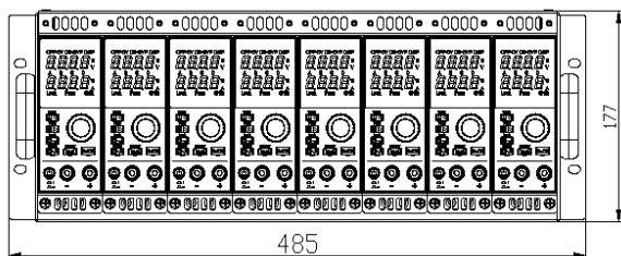
8路机箱尺寸（单位mm）
